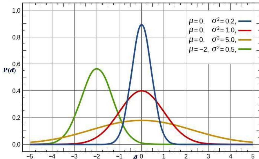
Σχήμα 2.4 Κανονική Κατανομή
